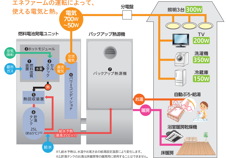
燃料電池発電ユニット (停電時自立発電機能付き) 192-AS11型
